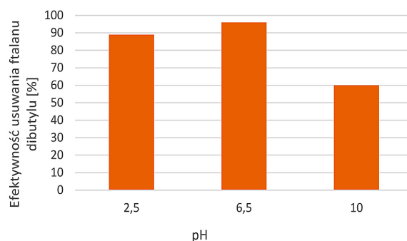
Rys. 4. Skuteczność usuwania ftalanu dibutyli przy zmiennym pH, czasie nadźwiękawiania t = 30 min i stałej amplitudzie drgań równej 20%
