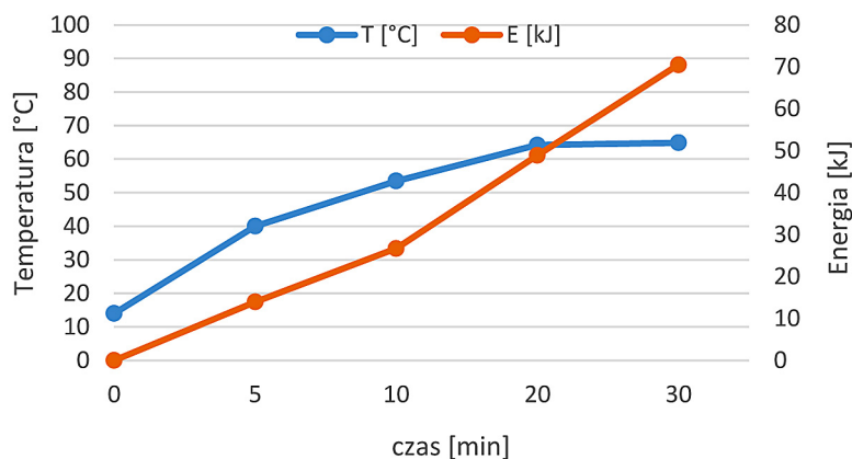
Rys. 5. Wpływ czasu nadźwiękawiania na zmianę temperatury oraz ilość wprowadzonej energii do próbek (amplituda 20%)
