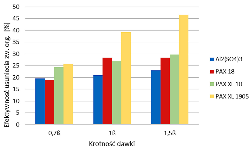
Rys. 2. Efektywność usuwania związków organicznych oznaczonych jako ChZT Cr w zależności od dawki oraz rodzaju koagulantu Fig. 2. The effect of the dose and type of coagulant on the effectiveness of COD removal
