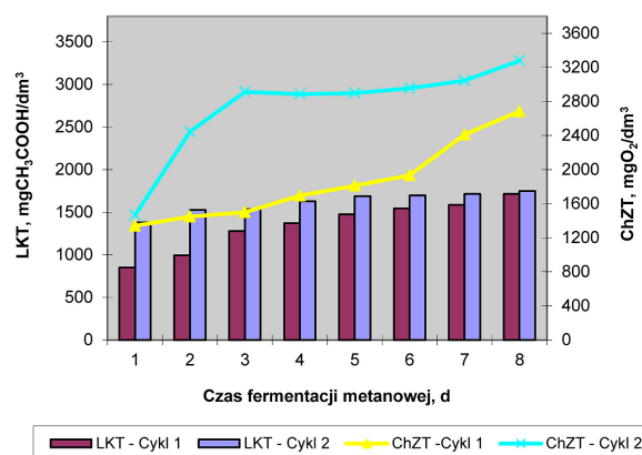
Rys. 2. Zmiany stężenia lotnych kwasów tłuszczowych i wartości chemicznego zapotrzebowania na tlen w kolejnych dniach termofilowej fermentacji metanowej w 1 i 2 cyklu badań
