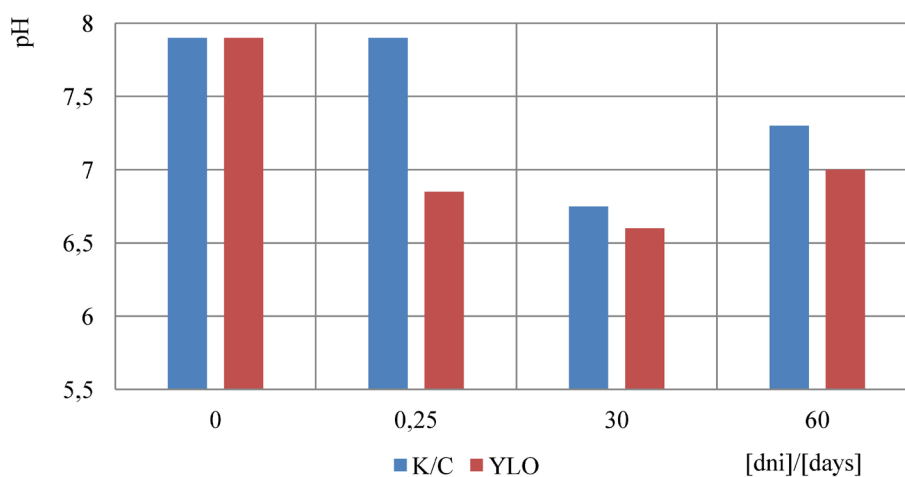
Rys. 2. Zmiany pH gleby skażonej substancjami ropopochodnymi po zastosowaniu techniki bioremediacji (K – kontrola; YLO – gleba stymulowana H_2O_2 i szczepionką Y. lipolytica A101)
