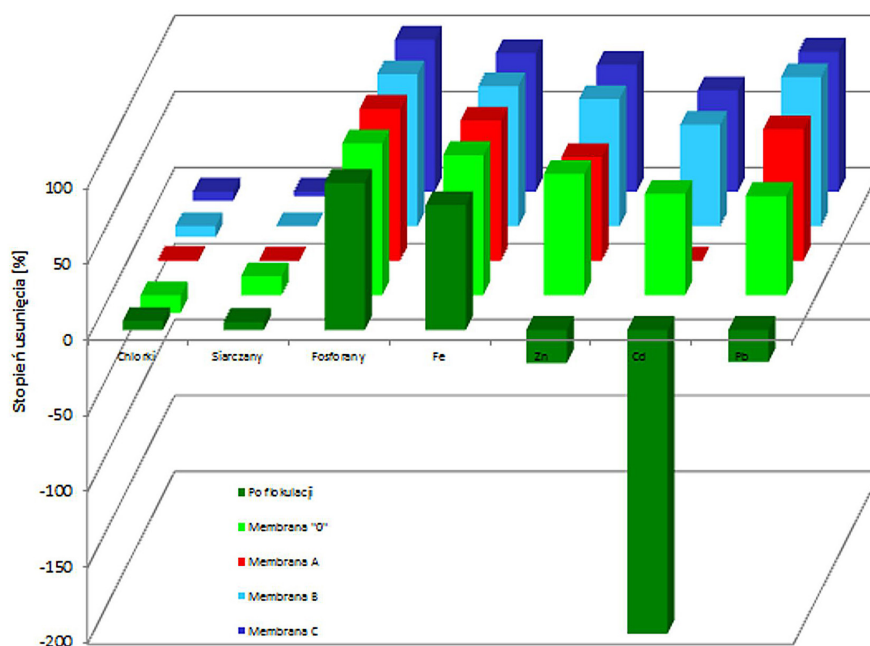
Rys. 6. Stopień usunięcia zanieczyszczeń w ściekach galwanizerskich po procesie flokulacji oraz ultrafiltracji Fig. 6. The degree of removal of pollutants in galvanic wastewater after flocculation and ultrafiltration processes
