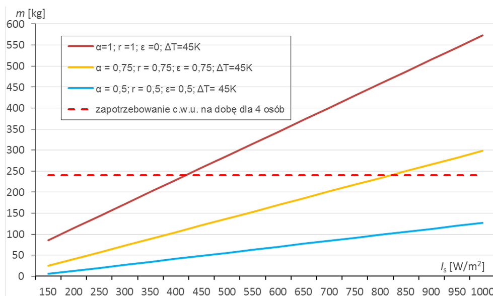
Rys. 5. Masa ogrzanej wody w czasie 6 godzin w zależności od strumienia promieniowania słonecznego dla zmiennych wartości parametrów \alpha , r , \varepsilon . Parametry przyjęte do obliczeń: w=1\text{m} , l=5\text{m} , T_c=328\text{K} , T_p=283\text{K} , ( \Delta T=45 ) i odpowiednio linia bordowa \alpha=r=1 , \varepsilon=0 , linia żółta \alpha=r=\varepsilon=0,75 , linia niebieska \alpha=r=\varepsilon=0,5 . Pozioma linia przerywana określa wydajność wynoszącą 240 litrów przy 6-godzinym oświetleniu promieniowaniem słonecznym, jest to zapotrzebowanie na c.w.u. dla czterech osób.
