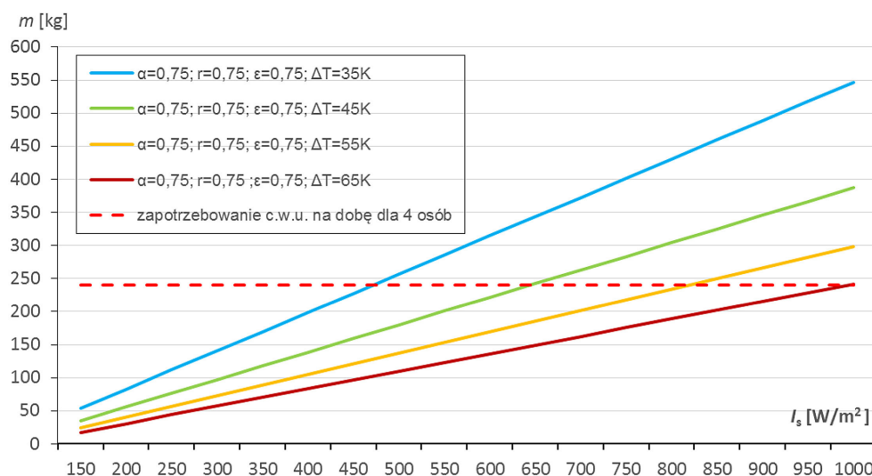
Rys. 6. Masa ogrzanej wody w czasie 6 godzin w zależności od strumienia promieniowania słonecznego dla różnych wartości temperatury końcowej wody użytkowej. Parametry przyjęte do obliczeń: w=1\text{m} , l=5\text{m} , przyjęto różnicę temperatur \Delta T=35\text{K} , \Delta T=45\text{K} , \Delta T=55\text{K} , \Delta T=65 współczynniki \alpha=r=\varepsilon=0,75 . Pozioma linia przerywana określa wydajność wynoszącą 240 litrów przy 6-godzinym oświetleniu promieniowaniem słonecznym, jest to zapotrzebowanie na c.w.u. dla czterech osób.
