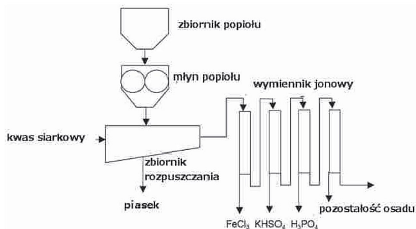
Rys. 6. Schemat procesu BIOCON [Levlin 2001, Poluszyńska i Ślęzak 2015]
